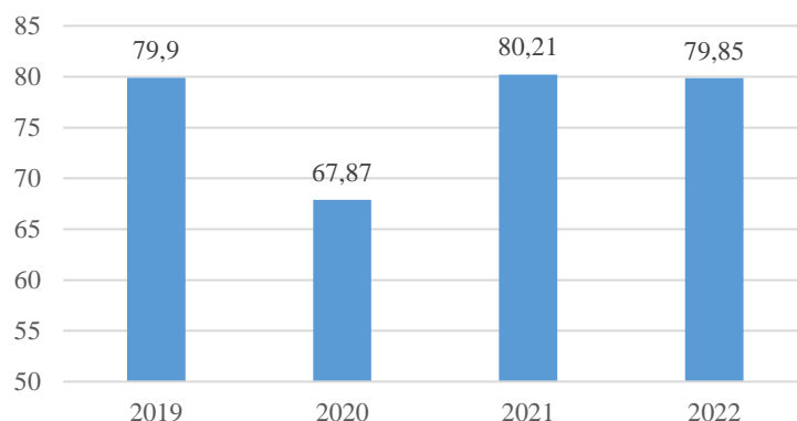
90. attēls. Vidējais īpatnējais izglītības iestāžu ēku siltumenerģijas patēriņš, kWh/m 2
