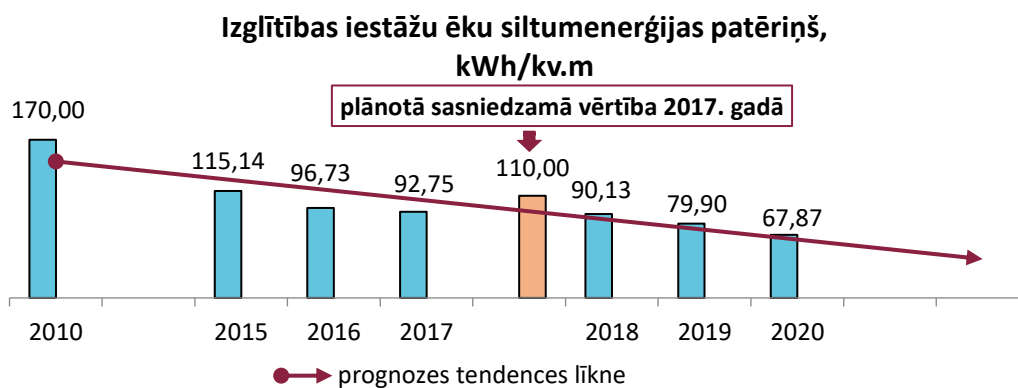
86. attēls. Izglītības iestāžu ēku siltumenerģijas patēriņa salīdzinājums
